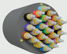
DETTAGLIO CAVO PICOBREAKOUT (altre colorazioni secondo tabella)
